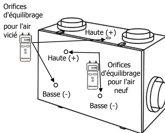
Vue d'ensemble des raccordements du débitmètre à hélice
