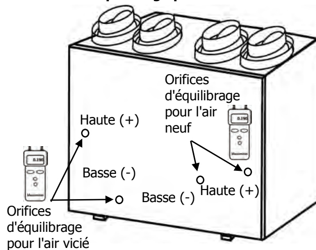
Vue d'ensemble des raccordements du débitmètre à hélice
